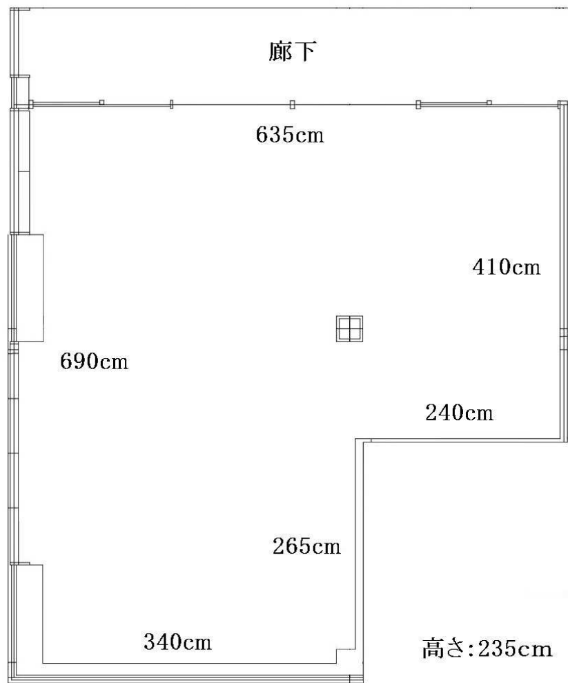
レンタルスタジオ平面図
